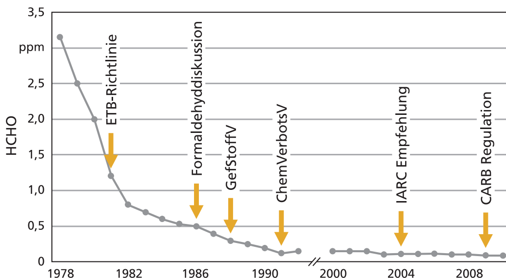
Abb. 7.3: Abnahme der Formaldehydabgabe von Holzspanplatten seit 1978
