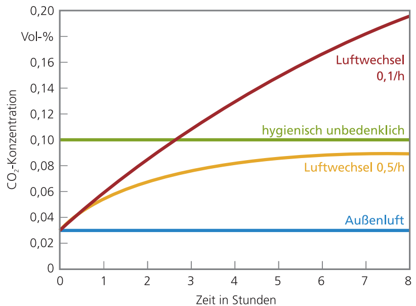
Abb. 6.1: Zunahme der \text{CO}_2 -Konzentration in einem 50 \text{ m}^3 Raum durch eine ruhende Person bei verschiedenen Luftwechselraten
