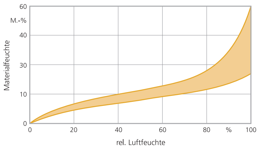
Abb. 5.4: Zusammenhang zwischen Materialfeuchte des Holzes und relativer Luftfeuchte
