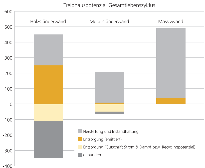
Abb. 4.3: Treibhauspotenzial verschiedener Innenwandtypen über den gesamten Lebensweg [Albrecht et al. 2008]
