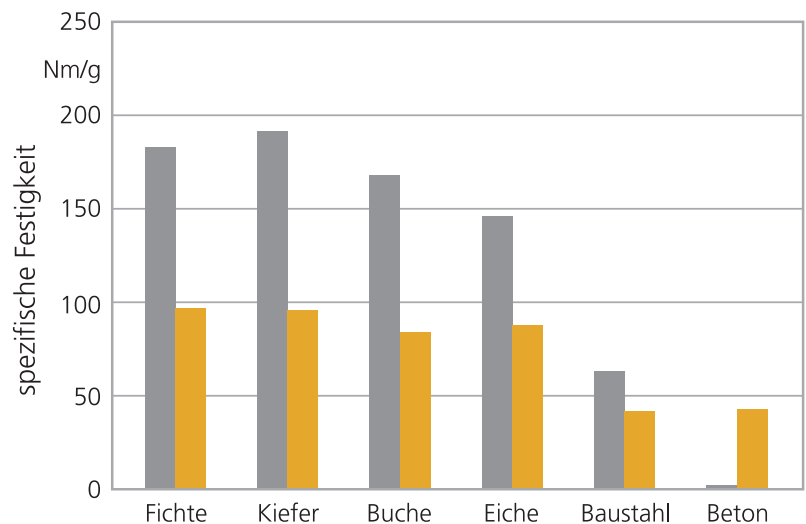
Abb. 2.3: Spezifische Zugfestigkeit (grau) und Druckfestigkeit (gelb) von einheimischen Hölzern im Vergleich zu Baustahl und Hochleistungsbeton
