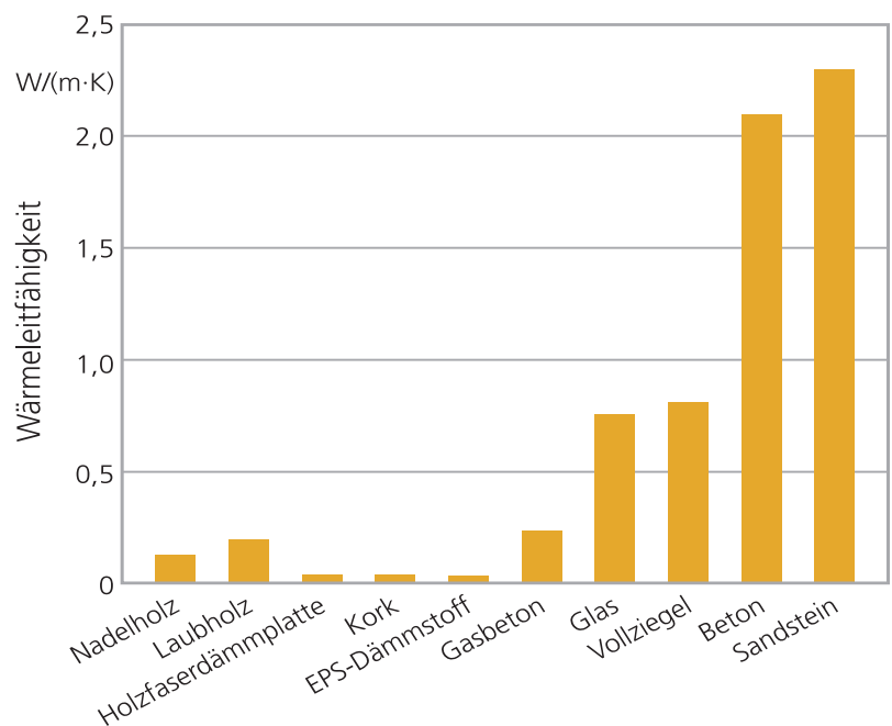
Abb. 9.1: Durchschnittliche Wärmeleitfähigkeiten einiger Dämm- und Baustoffe
