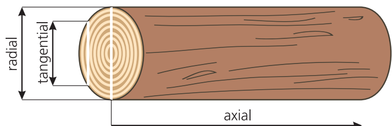
Abb. 2.2: Darstellung der drei Grundrichtungen von Holz
