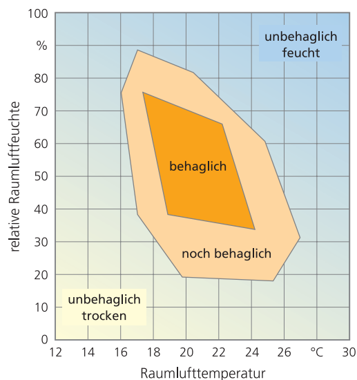
Abb. 5.3: Behaglichkeitsdiagramm für die Raumluftparameter Temperatur und Luftfeuchte
